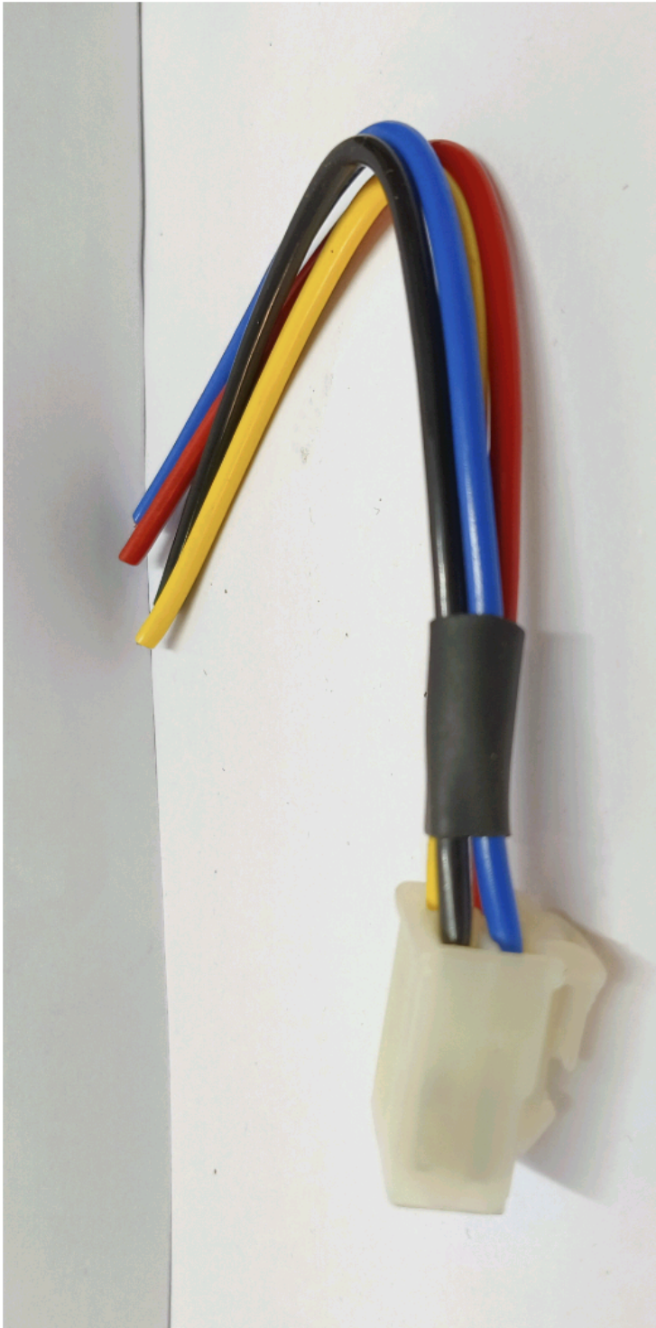
Brake Switch coupler N/M(4 wire)
